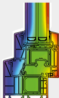
Průběh izoterm
