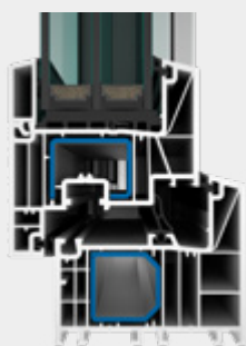
Uzavřená ocelová výztuha v rámu a ocelová výztuha křídla
