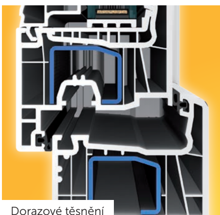
Dorazové těsnění
